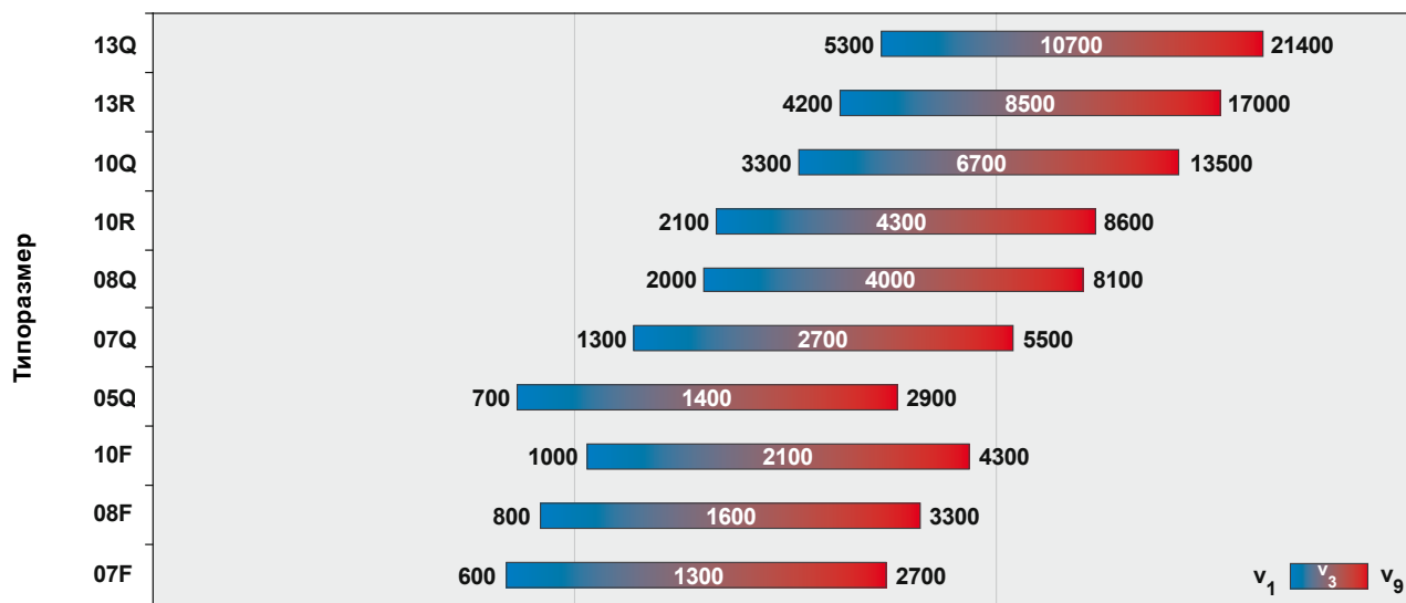
Производительность (м³/ч)
