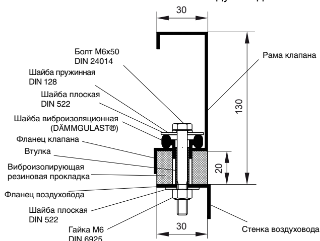
На чертеже показан узел соединения воздушного клапана в гигиеническом исполнении и воздуховода:
