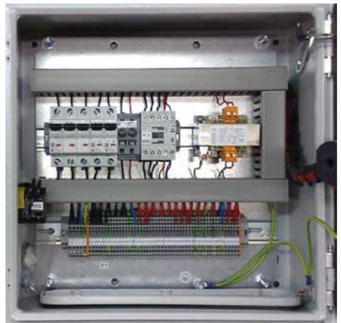
Примерное изображение аппаратуры управления «MSD-TR»
